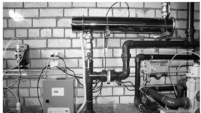
UV-steriliseerimisseade
