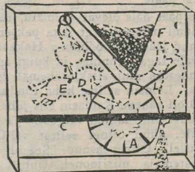
Joon. 6. Liivatsirkuse mehanism (tagantvaade).
