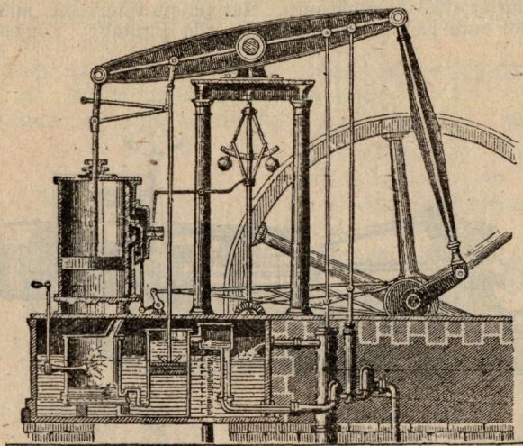
Aurumasin (sisemüüritud).
