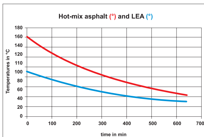
Joonis. Kuuma asfaltbetooni (°C) ja LEA (°C) temperatuurigradiendide võrdlus
