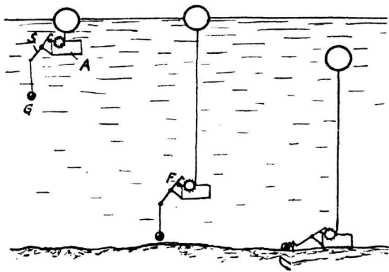
Joon. 3. Üks miiniveeskmise mooduseid
