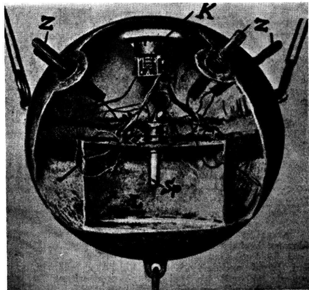
Joon. 1. Vene sarvmiin läbilõikes
