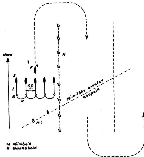
Joon. 5. Miinide traalimine
