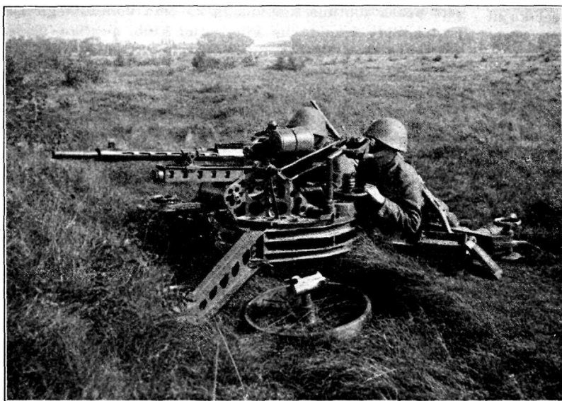
Daani „Madsen'i“ 20 mm kahur ratastelt mahavõetuna
