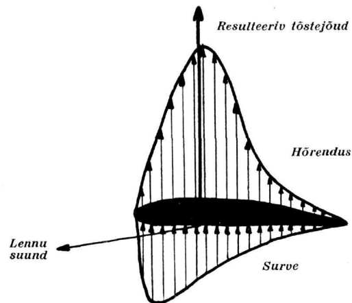
Joon. 11. Õhusurve muutlikkus profiili sügavust mööda
