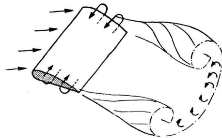
Joon. 15. Keeriste tekkimine tiiva otstel
