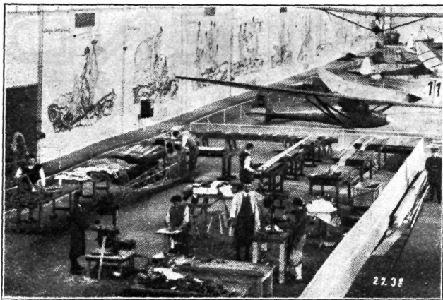
Purilennukite ehituse töökoda „Dela“ näitusel Berliinis. Tagaplaanil ins. Bachem'i kõrgeväärtuslik rekordpurilennuk „Termikus“, mille valmistanud Stuttgart'i akadeemiline lennuseelts 5000 töötunniga
