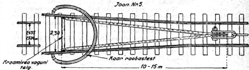
Joan. Nr. Nr. 4 ja 5 - teepurustajad, missuguseid kasutati Koléaki armees.
