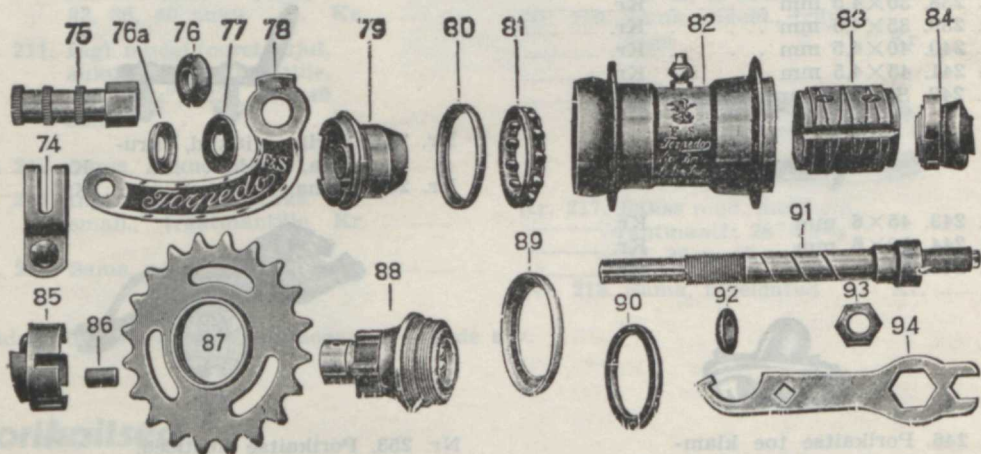
Nr. 261. Torpedo rumm kpl., nikeld. 66 ja 40 auku . . . . . Kr. ....
