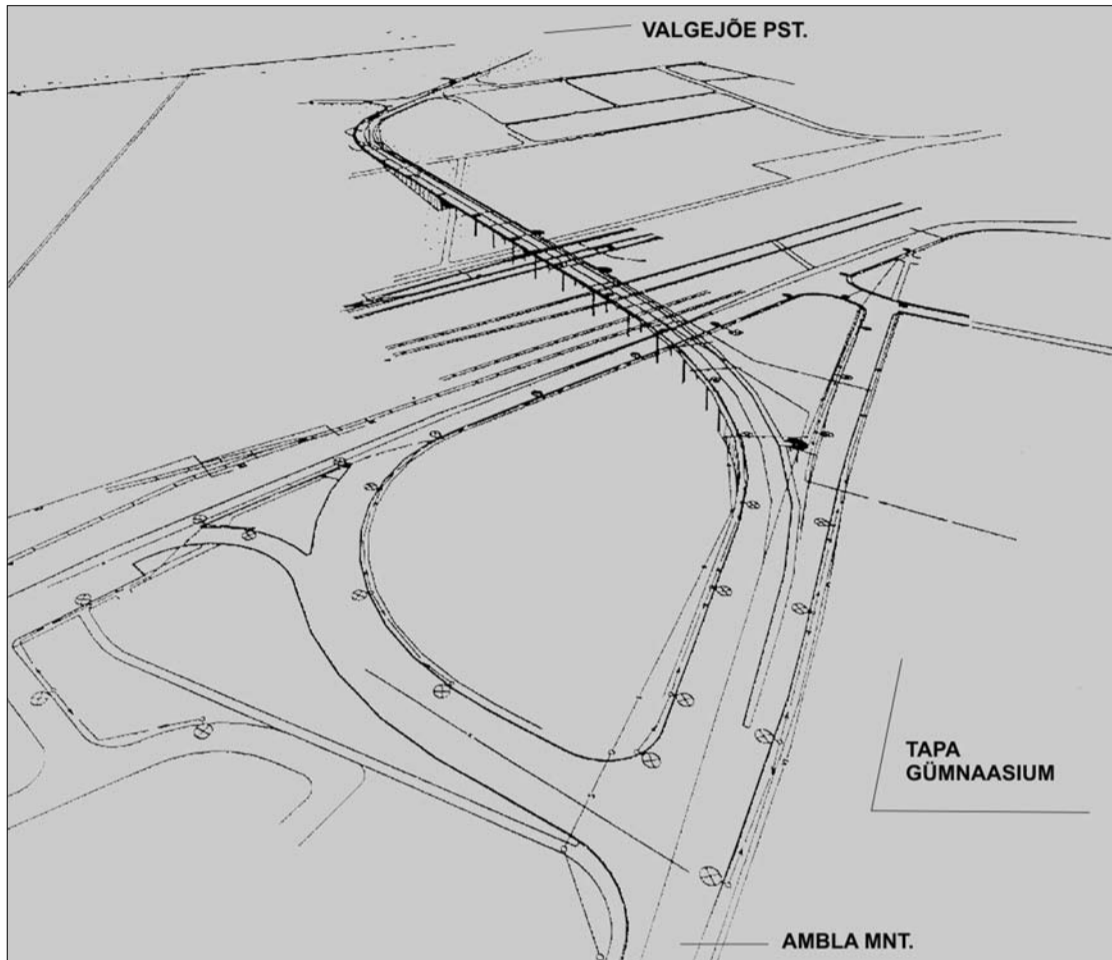
Рабочий рисунок из проекта будущего виадука, разработанный на первом этапе проектирования.
