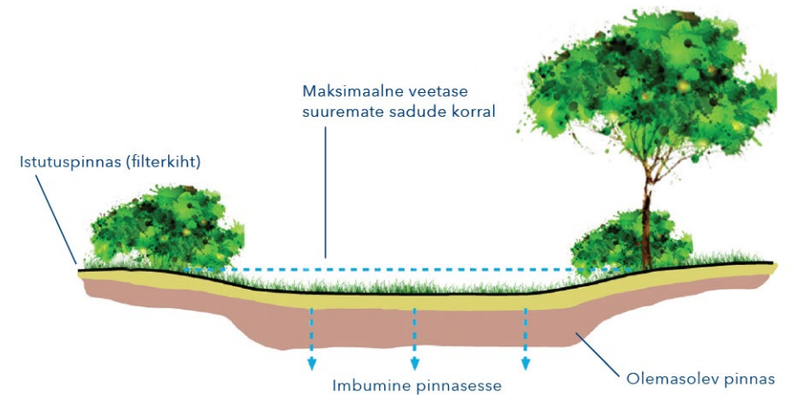
Joonis 12. Viibetiigi läbilõige.
