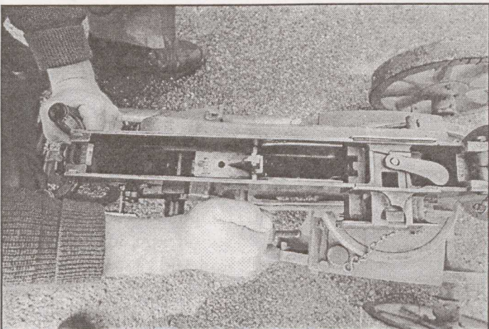
Lukk on vinnas. Päästikule vajutusel liigub lukk ette, suunab padrundi rauda ja toimub lask. Vända käepide kordab iga lasu järel vinnastamiseks vajalikku liikumist.
