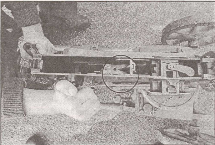
Vinnastusvända käepidet ette lükates liigub lukk mööda lukukoja karbisooni tahapoole.
