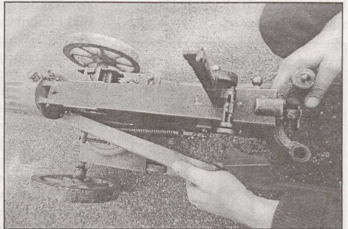
Kuulipilduja pealtvaade avatud taandurvedru karbiga.
