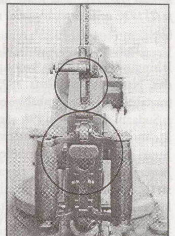
Kuulipilduja tagantvaates. Ülal reguleeritav sihik, all käepidemed, keskel päästik koos selle kohal asetseva kaitseriiviga.
