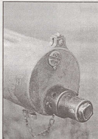
Rauasudmel olev gaasikamber suunab lasu järel raua tagasi, mille toimel lukumehhanism valmistab relva ette järgmiseks lasuks.
