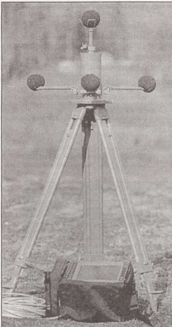
Kanadas valmistatud Guardiani komplekti kuuluvad kolmjalgjel statiivil asetsev mikrofonid ja analüüsiseade.
