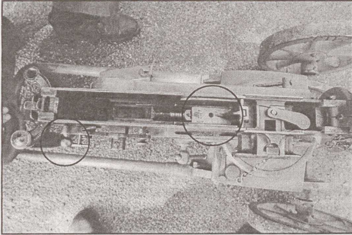
Kuulipilduja avatud lukukojaga. Lukk on eesendis, vinnastusvända käepide on algasendis.
