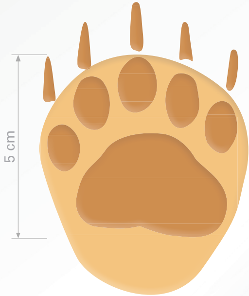
Parem esikäpp
