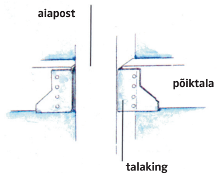
Joonis 3. Põiktalade kinnitamine postide külge
