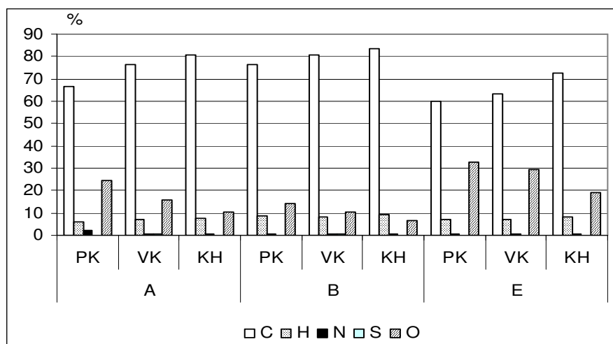
Joonis 3. Koorest poolkoksistamisel (PK), vesikonversioonil (VK) ja katalüütilisel hüdrogeenimisel (KH) saadud õlide atsetooni- (A), benseeni- (B) ja eetriekstraktide (E) elemendikoostis %
