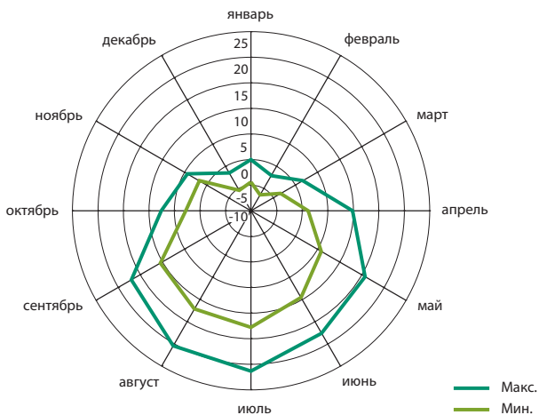
Средняя максимальная и минимальная температура воздуха, 2009
