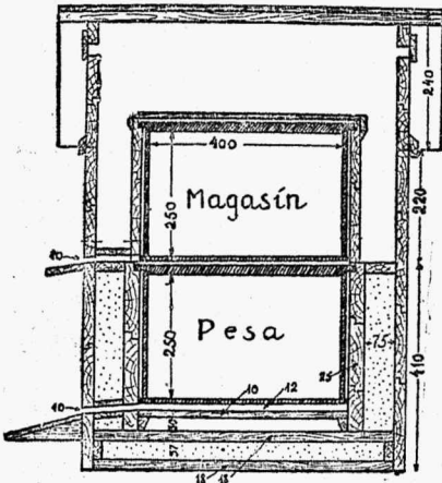
Joon. 2. Püstlülilõige.
