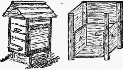
Joon. 1. Eesti taru. Joon. 3. A, B, C — siseseinad, D — põhi, E — välissein ja F — pidekliistud.
