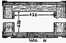
Joon. 4. Ristlülilõige.
