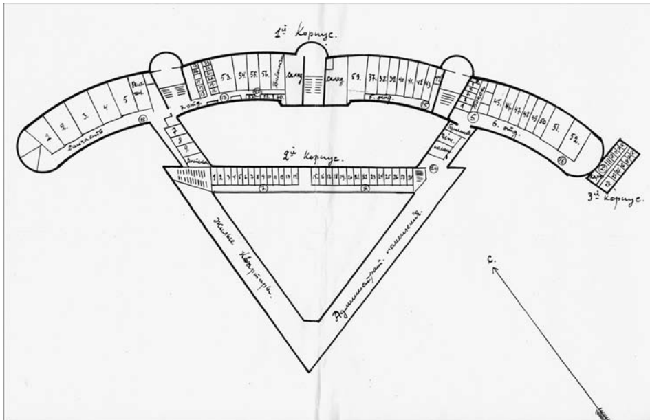
Keskvangla 2. korruse skeem: 1. korpus (vana merekindlus), 2. korpus (ehitati 1935) ja 3. korpus (ehitati 1931). Arhiivi dokument [29, l. 12].
