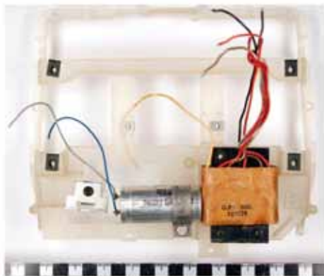
Lauakalkulaatori korpus, millest pool leiti sündmuskohalt ning teine pool neli ja pool aastat hiljem Ringmaa kodust.
