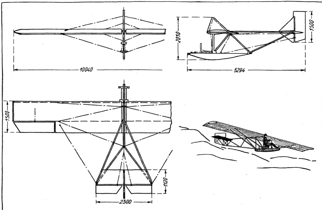
Purilennuki osade koostamise joonis Mõõt: 1:50.
