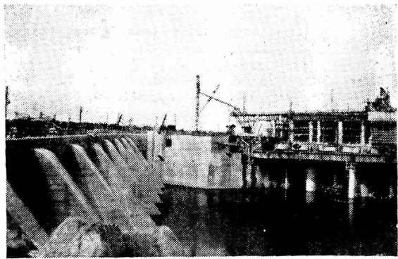
Ehitatav hiigel-elektrijõujaam Düüna jõel, 40 km Riüst
