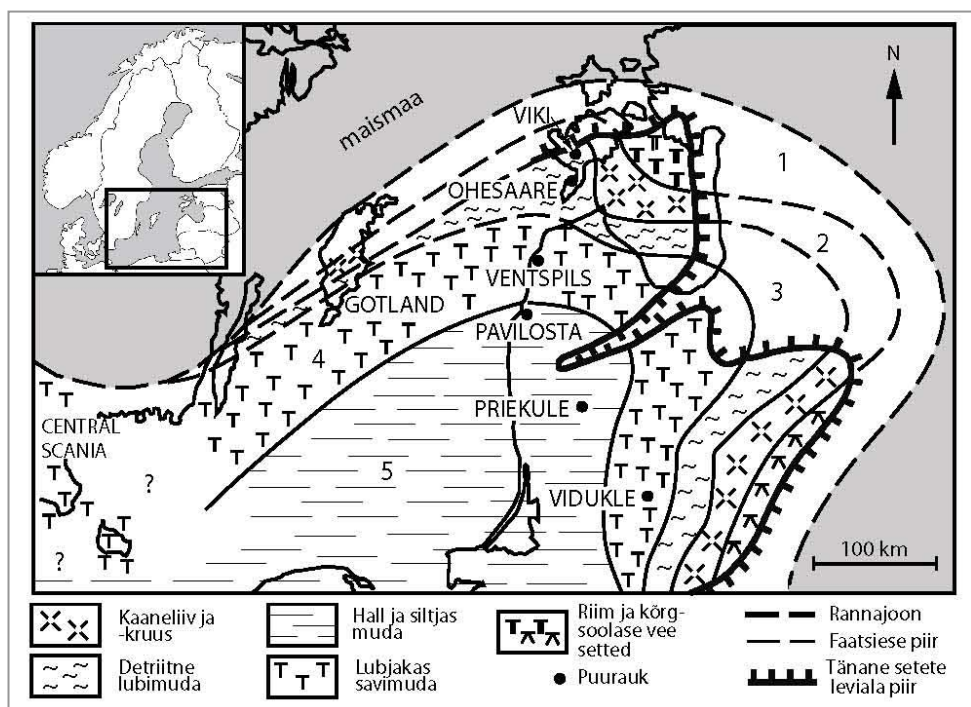
Joonis 1. Balti basseini faatsieste levik Ludlow ajastiku alguses (modifitseeritud Bassett jt 1989 järgi) ja uuritud puursüdame asukohad. Faatsieste vööndid: 1. Tõusu-mõõna ala ja laguunid. 2. Madalikud ja tugeva lainetuse ala. 3. Avašelf. 4. Süvašelf. 5. Šelfi depressioon ja üleminek avamerele.
