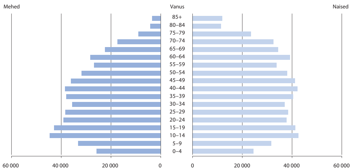
Rahvastiku vanuspüramiid, 2000
