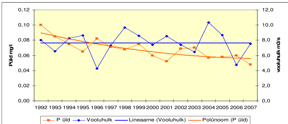
Joonis 1.8. Riikliku seireprogrammi jõgede üldfosfori ja hüdroloogilistes vaatluspostides mõõdetud vooluhulkade (välja arvatud Narva jõgi) aastakeskmised väärtused
