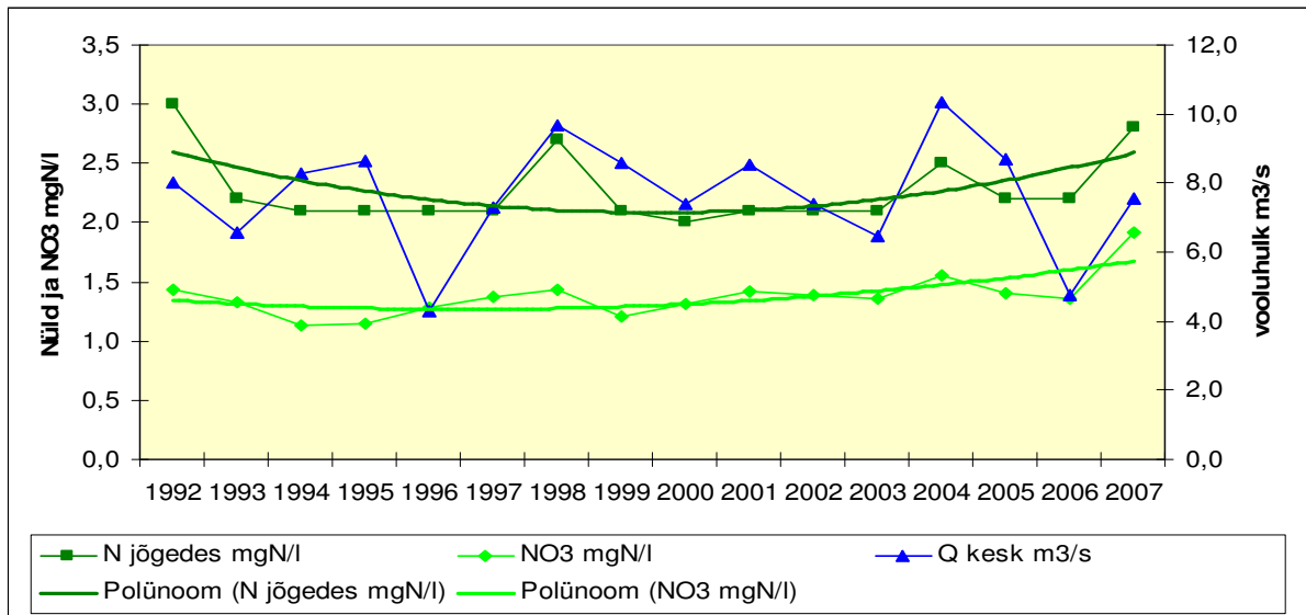
Joonis 1.7. Riikliku seireprogrammi jõgede üld- ja nitraatlämmastiku ning hüdroloogilistes vaatluspostides mõõdetud vooluhulkade (välja arvatud Narva jõgi) aastakeskmised väärtused
