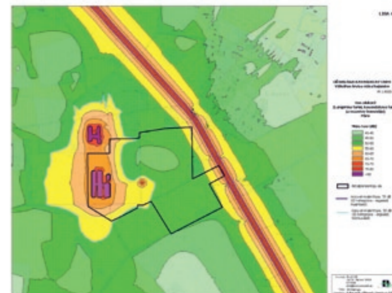
Joonis 2. Rajatava objekti ja maantee koostõu. Müra tase prognoos päeval
