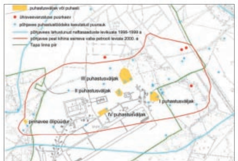
Jaanis 40 Tapa lennuvälja reovärskelle ja põhjavee puhastustööde väljakul
