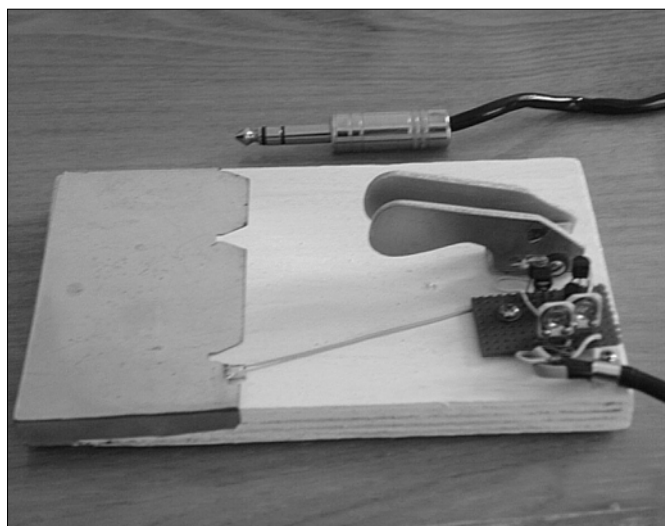
Sensormanipulaator valmiskujul
