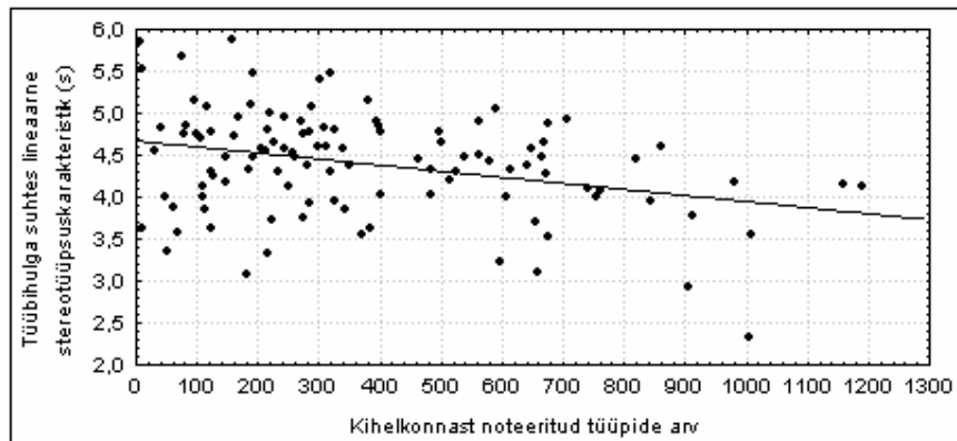
Joon. 10. Lineaarne stereotüüpsuskarakteristik s_K
