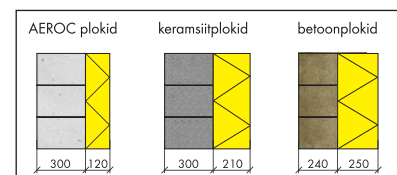
Passiivmaja ökonoomsem lahendus – AEROC sein
