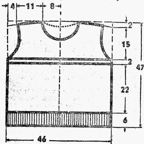
Joon. 4. Heegelpuusi lõige.
