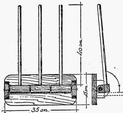
Joon. 2. Püstloodis liikuvate pulkadega käteräti hoidja.
