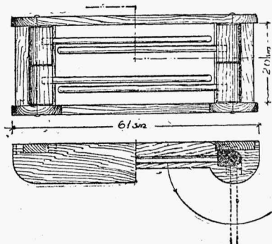
Joon. 1. Liikuvate pulkadega käteräti hoidja.
