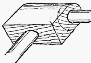
Joon. 3. Liikuv klot.
