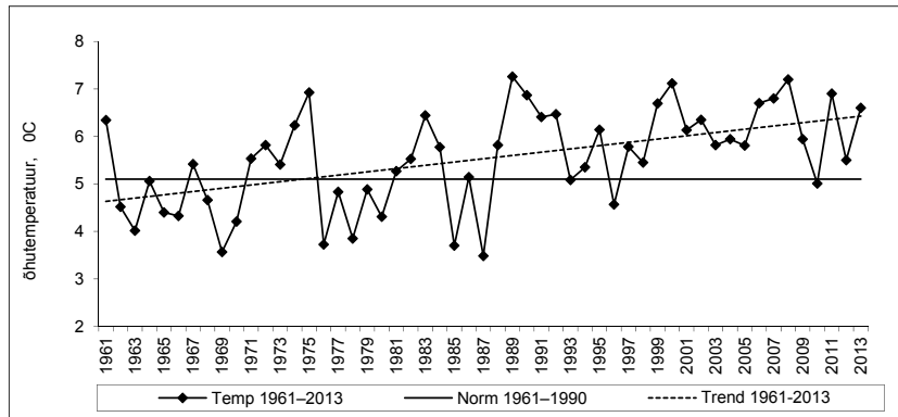
Joonis 5-2. Valga aasta keskmise õhutemperatuuri (°C) aegrida 1961–2013
