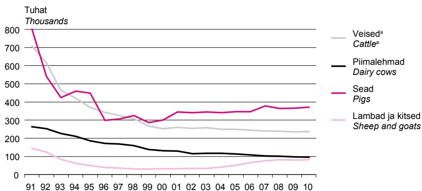
Joonis 1. Loomad, 1991–2010
