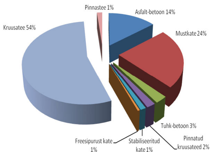
Joonis 7-37 Riigiteede katted
