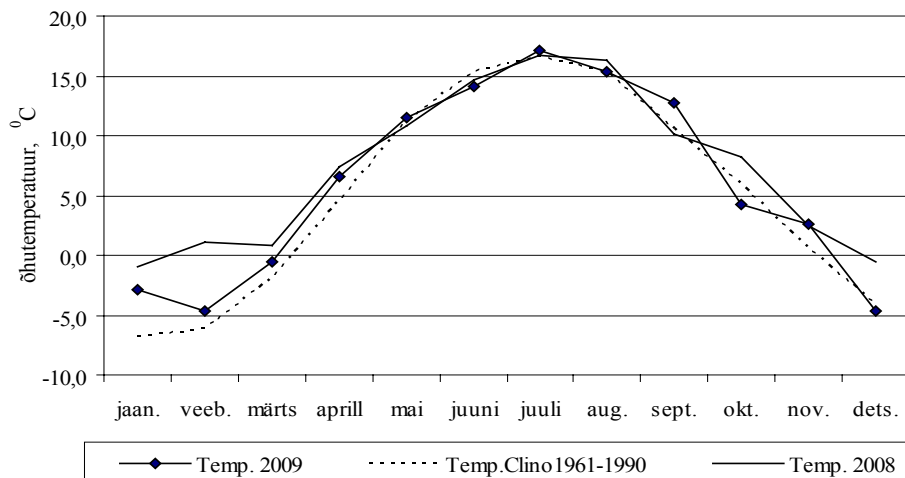
Joonis 5-3 Valga. Kuu keskmine õhutemperatuur (°C)
