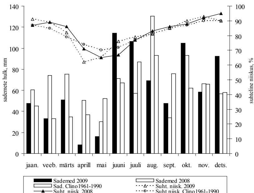
Joonis 5-4 Valga. Sademete hulk, mm ja suhteline õhuniiskus, %
