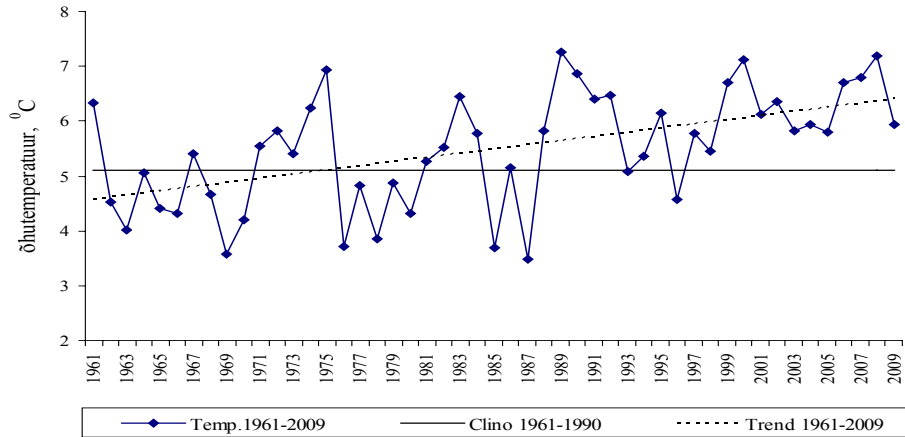
Joonis 5-2 Valga. Aasta keskmise õhutemperatuuri (°C) aegrida
