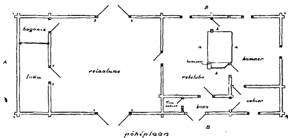
põhiplaan
