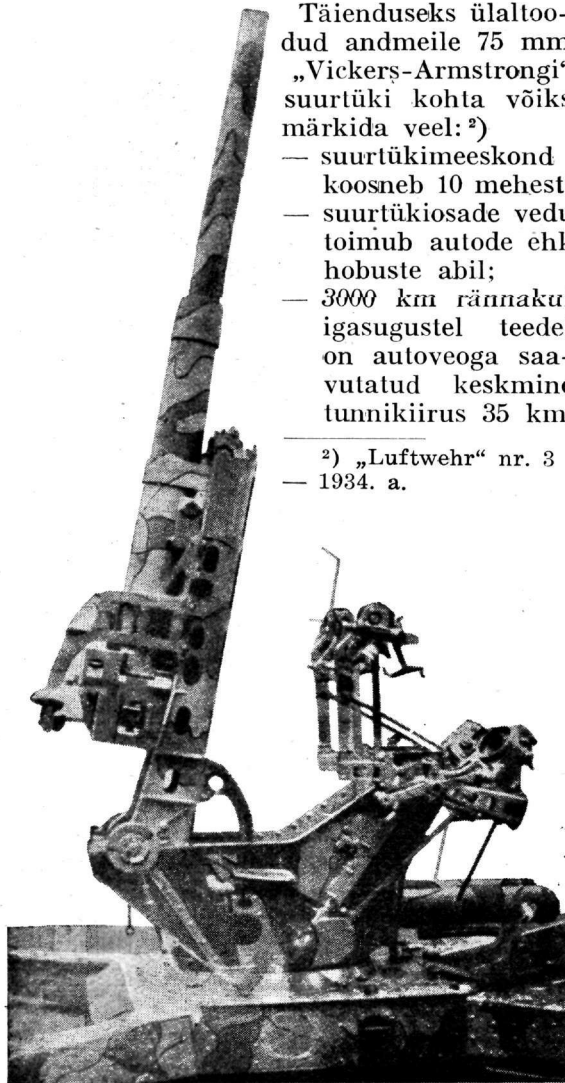
Pilt nr. 1. „Vickers-Armstrong“ 75 mm õhk-kahur.
