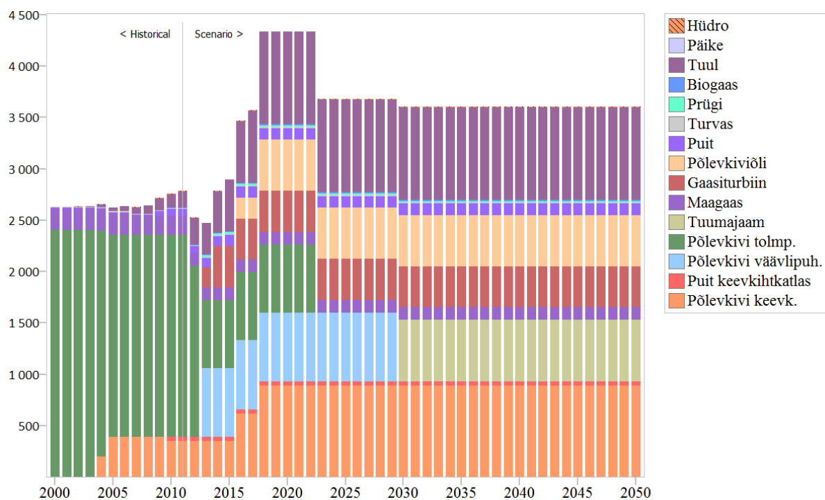
Joonis 126. BAU stsenaariumi elektri tootmisvõimsused, MW.
