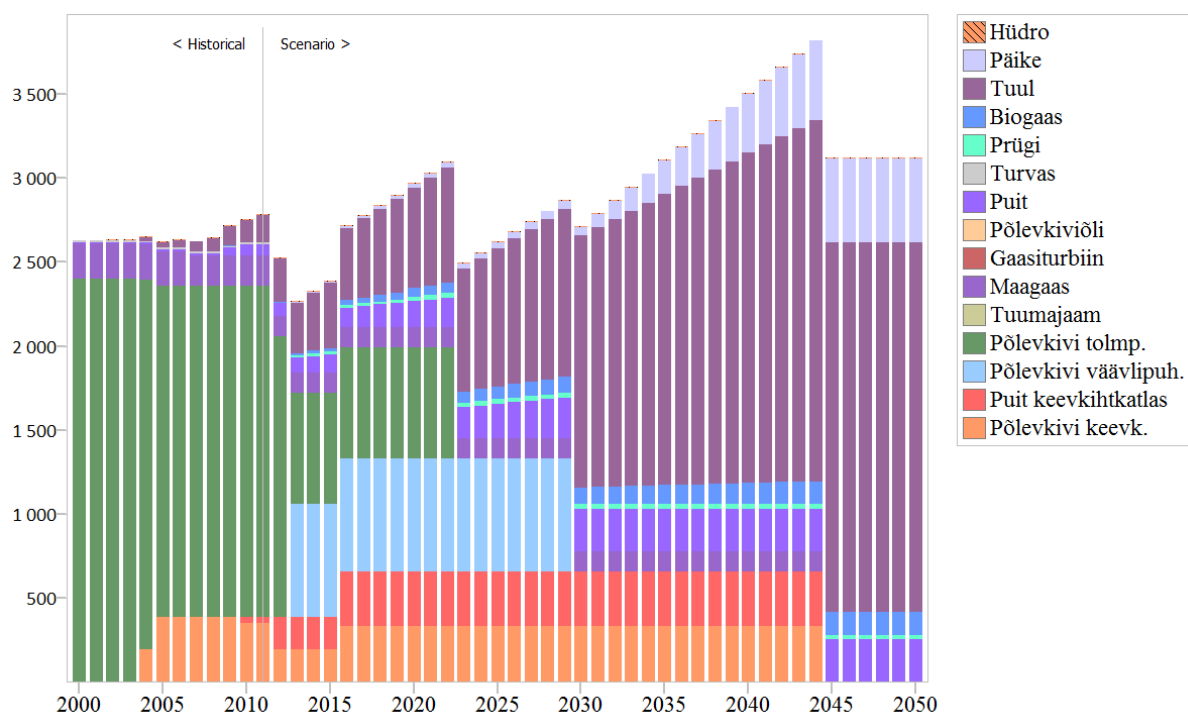
Joonis 128. LOW CO2 stsenaariumi elektri tootmisvõimsused, MW.
