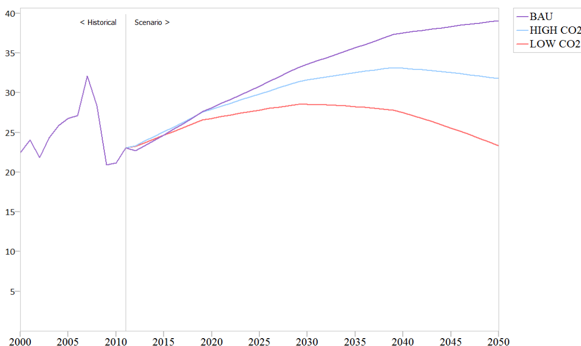
Joonis 23. Energia lõpptarbimise prognoos töötlevas tööstuses, tuhat TJ.
