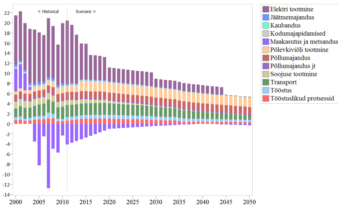
Joonis 86. Stsenaariumi Madalsüsinik KHG heitkogused, mln t.
