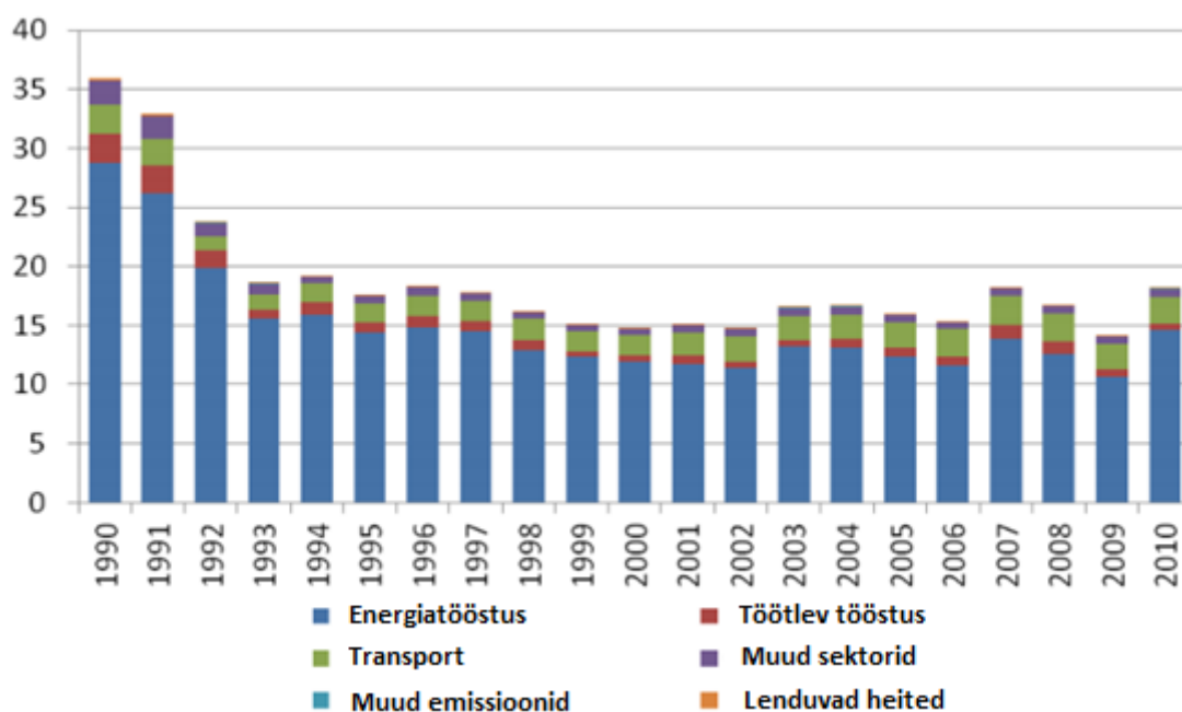
Joonis 2. Energiamaajanduse sektori KHG heide välisõhku aastatel 1990–2010, mln t CO 2 -ekv.
