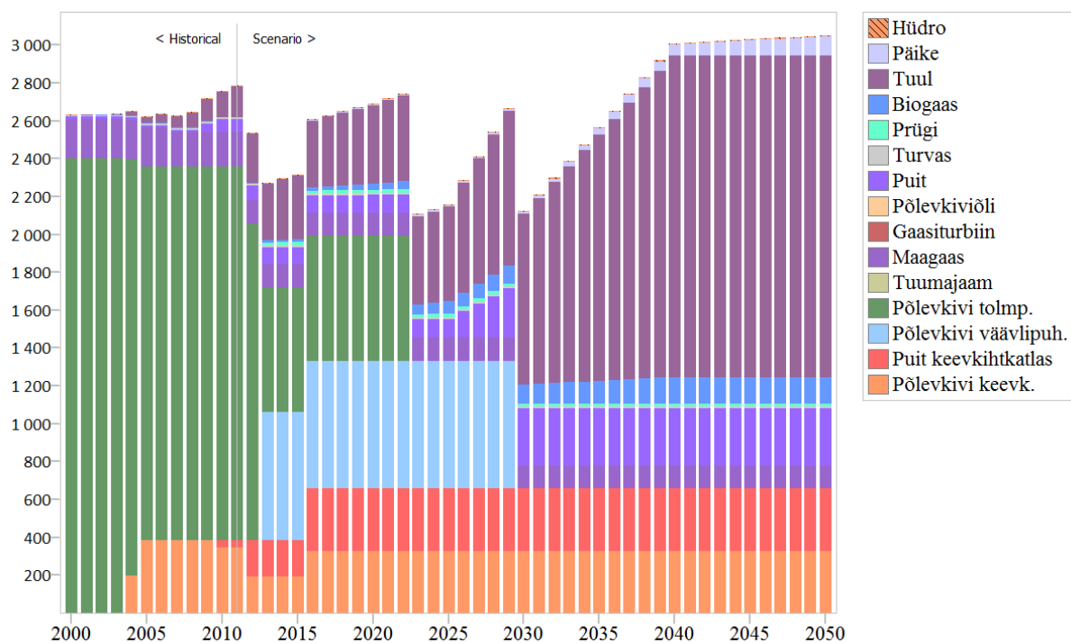
Joonis 127. HIGH CO2 stsenaariumi elektri tootmisvõimsused, MW.
