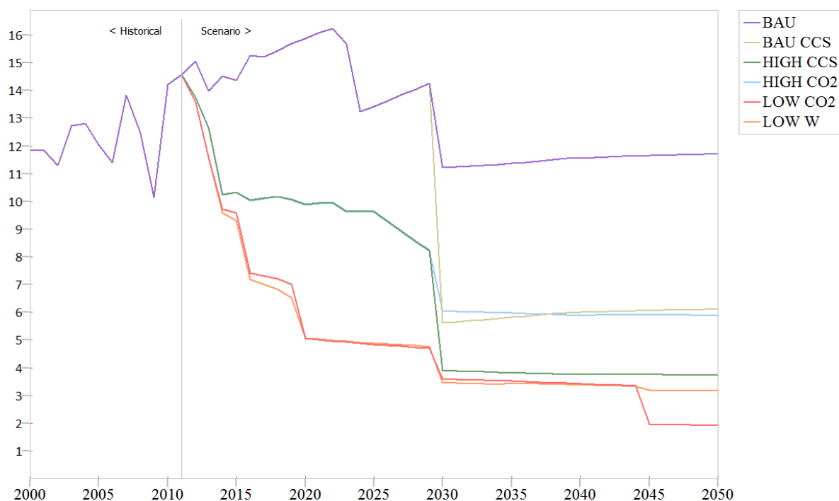
Joonis 38. Energiatööstuse (elektri, soojuste ja põlevkiviõli tootmise) KHG heitkoguste prognoos.
