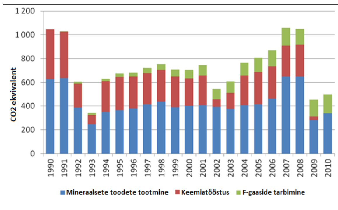
Joonis 53. Tööstuslike protsesside KHG heitkogused Eestis perioodil 1990–2010, tuhat tonni CO 2 -ekv.
