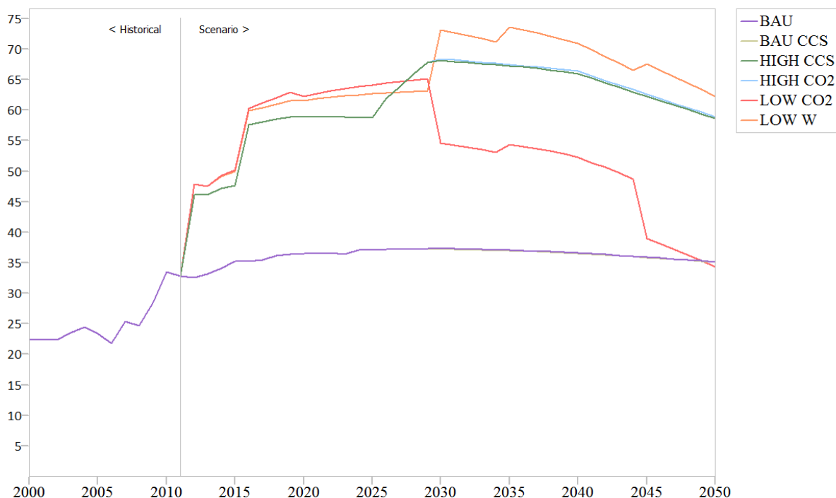
Joonis 30. Energiamaanduse puidu tarbimismahutude prognoos, tuhat TJ.
