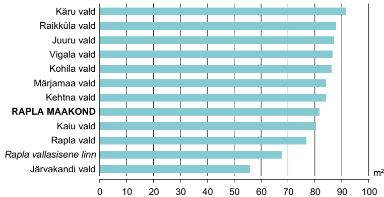
Joonis X-34. Tavaeluruumide keskmine suurus Rapla maakonna valdades, 31.12.2011
