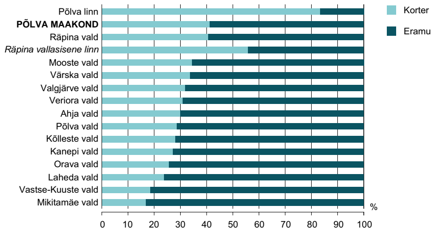
Joonis VIII-35. Põlva maakonna linnade ja valdade tavaeluruumide struktuur, 31.12.2011
