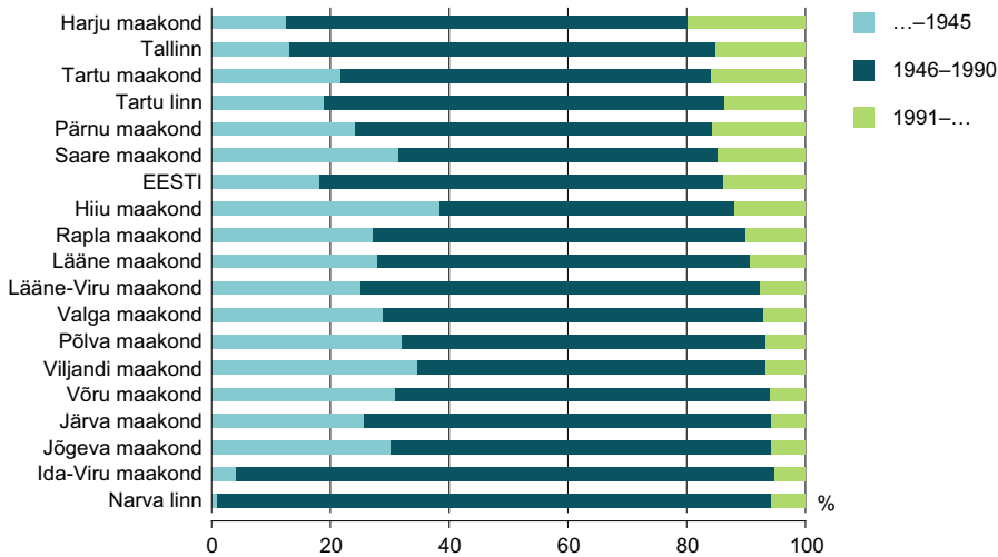
Joonis 7.3. Tavaeluruumid maakondades ja suurtes linnades ehitusaja järgi, 31.12.2011
