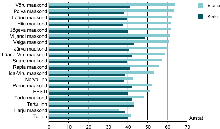
Joonis 7.4. Maakondade ja suurte linnade tavaeluruumid keskmise hinnangulise vanuse järgi, 31.12.2011
