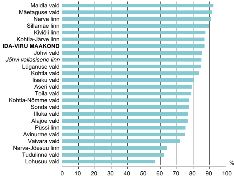
Joonis III-38. Ida-Viru maakonna linnade ja valdade tavaeluruumide asustatus, 31.12.2011
