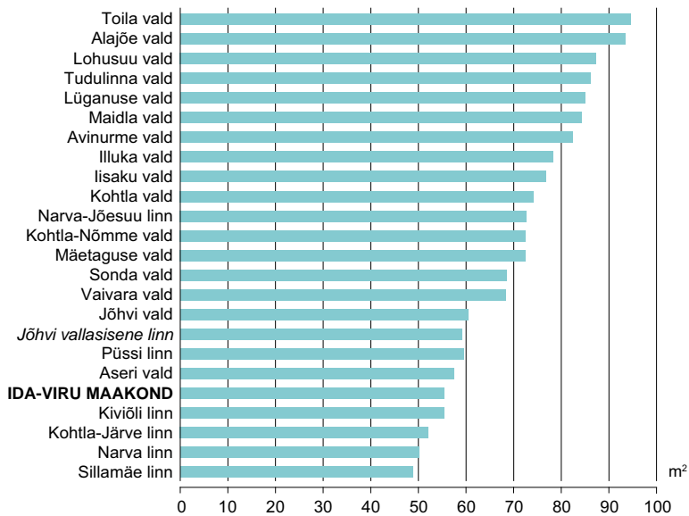
Joonis III-34. Tavaeluruumide keskmine suurus Ida-Viru maakonna linnades ja valdades, 31.12.2011
