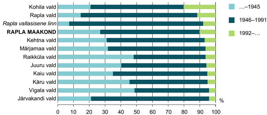
Joonis X-37. Rapla maakonna valdade tavaeluruumidega hooned ehitusaja järgi, 31.12.2011
