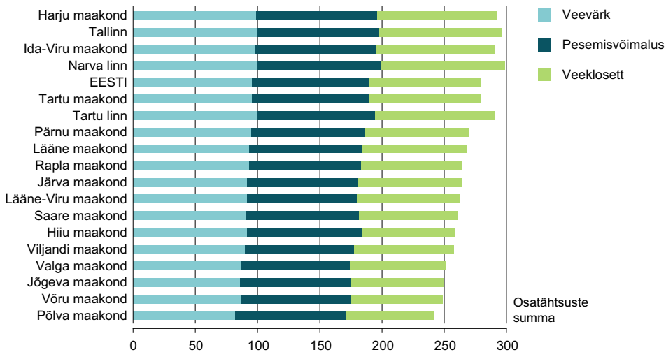
Joonis 7.13. Maakondade ja suurte linnade elanikud veevärki, pesemisvõimaluse ja veekloseti olemasolu järgi eluruumis, 31.12.2011
