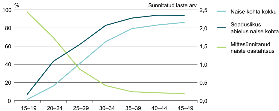
Joonis VII-32. Lääne-Viru maakonna naiste keskmine sünnitatud laste arv ja mittedünnitanud naiste osatähtsus vanuserühma järgi, 31.12.2011
