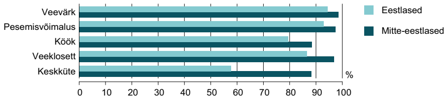
Joonis 7.14. Tavaeluruumide tehovarustus elanike rahvuse järgi, 31.12.2011
