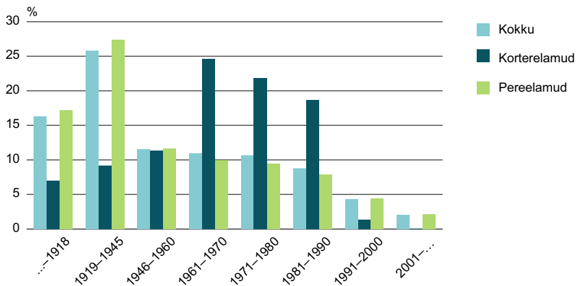
Joonis IV-36. Jõgeva maakonna tavaeluruumidega hooned ehitusaja ja hoone tüübi järgi (osatähtsus sama tüüpi hoonete hulgas), 31.12.2011
