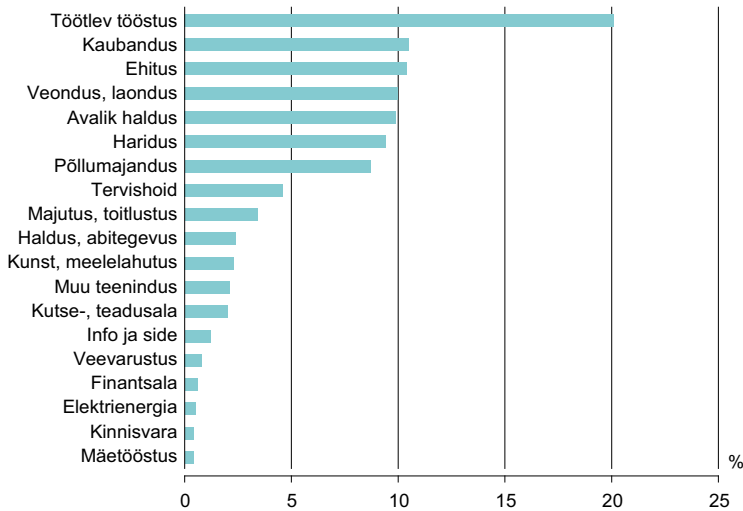
Joonis II-27. Vähemalt 15-aastased Hiiu maakonna töötajad tegevusala järgi, 31.12.2011
