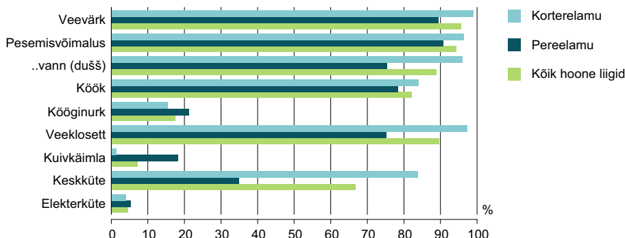
Joonis 7.11. Korter- ja pereelamud tehnovarustuse järgi, 31.12.2011
