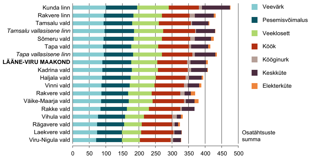
Joonis VII-39. Lääne-Viru maakonna linnade ja valdade tavaeluruumid tehnavarustuse järgi, 31.12.2011
