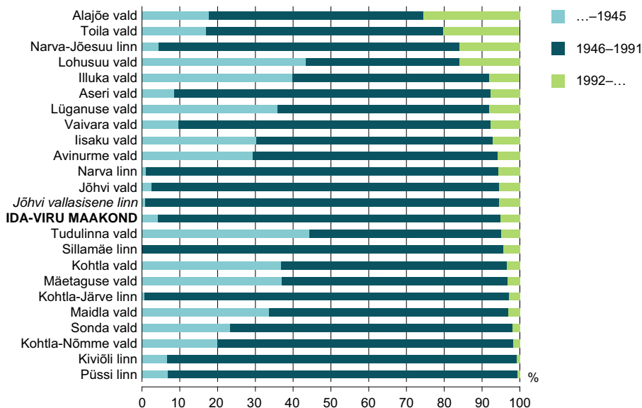
Joonis III-37. Ida-Viru maakonna linnade ja valdade tavaeluruumid ehitusaja järgi, 31.12.2011
