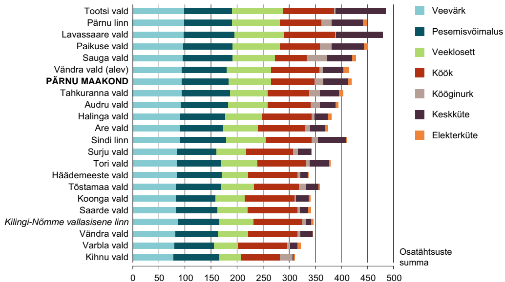
Joonis IX-39. Pärnu maakonna linnade ja valdade tavaeluruumid tehnovarustuse järgi, 31.12.2011
