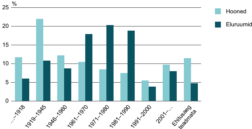
Joonis 7.2. Elamiskõlblikuna säilinud hooned ja eluruumid ehitusaja järgi (osatähtsus kõrgis loendatud tavaeluruumidega hoonetes, neis asuvates eluruumides), 31.12.2011
