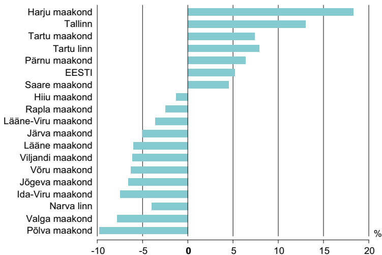
Joonis 7.1. Maakondade ja suurte linnade tavaeluruumide arvu muutus, 31.03.2000–31.12.2011
