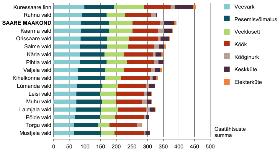
Joonis XI-39. Saare maakonna Kuressaare linna ja valdade tavaeluruumid tehnavarustuse järgi, 31.12.2011
