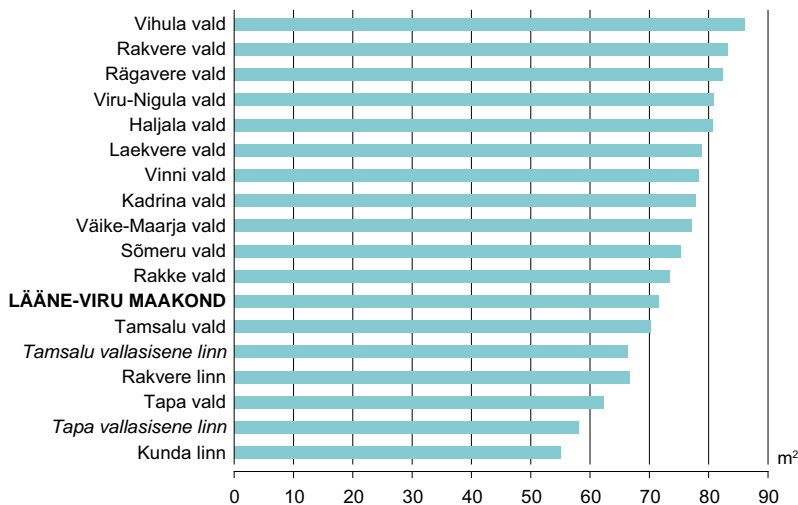
Joonis VII-34. Tavaeluruumide keskmine suurus Lääne-Viru maakonna linnades ja valdades, 31.12.2011
