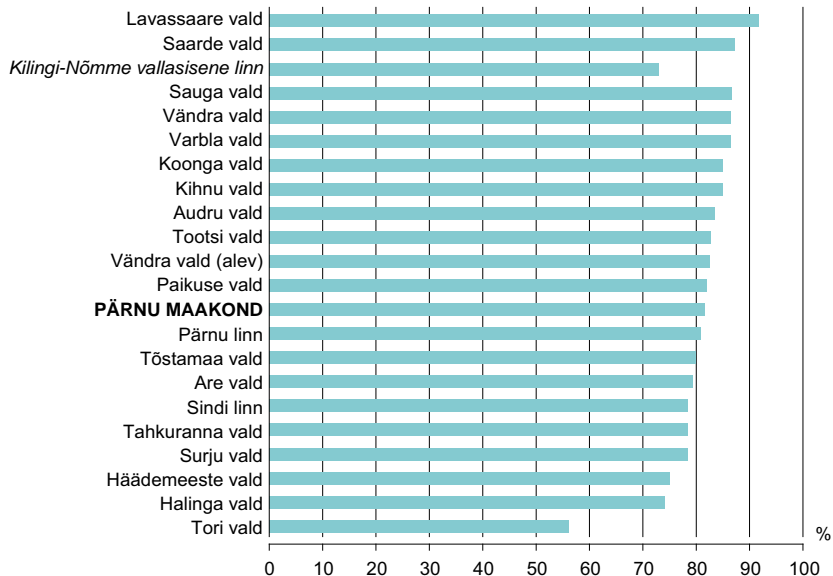
Joonis IX-38. Pärnu maakonna linnade ja valdade tavaeluruumide asustatus, 31.12.2011
