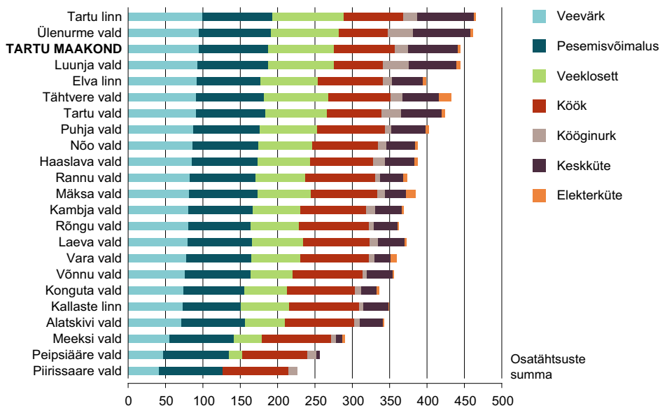
Joonis XII-39. Tartu maakonna linnade ja valdade tavaeluruumid tehnovarustuse järgi, 31.12.2011
