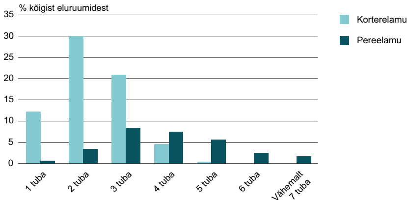
Joonis 7.9. Korter- ja pereelamud tubade arvu järgi, 31.12.2011
