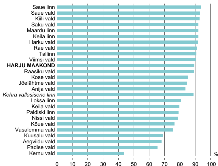
Joonis I-38. Harju maakonna linnade ja valdade tavaeluruumide asustatus, 31.12.2011
